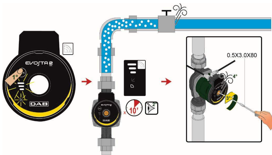
Obrázek 16: Odvzdušnění čerpadla
