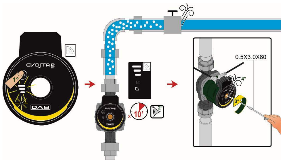
Obrázok 16: Odvzdušnenie čerpadla
