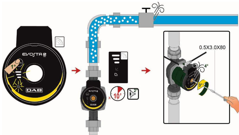
Abb 16: Pumpentlüftung
