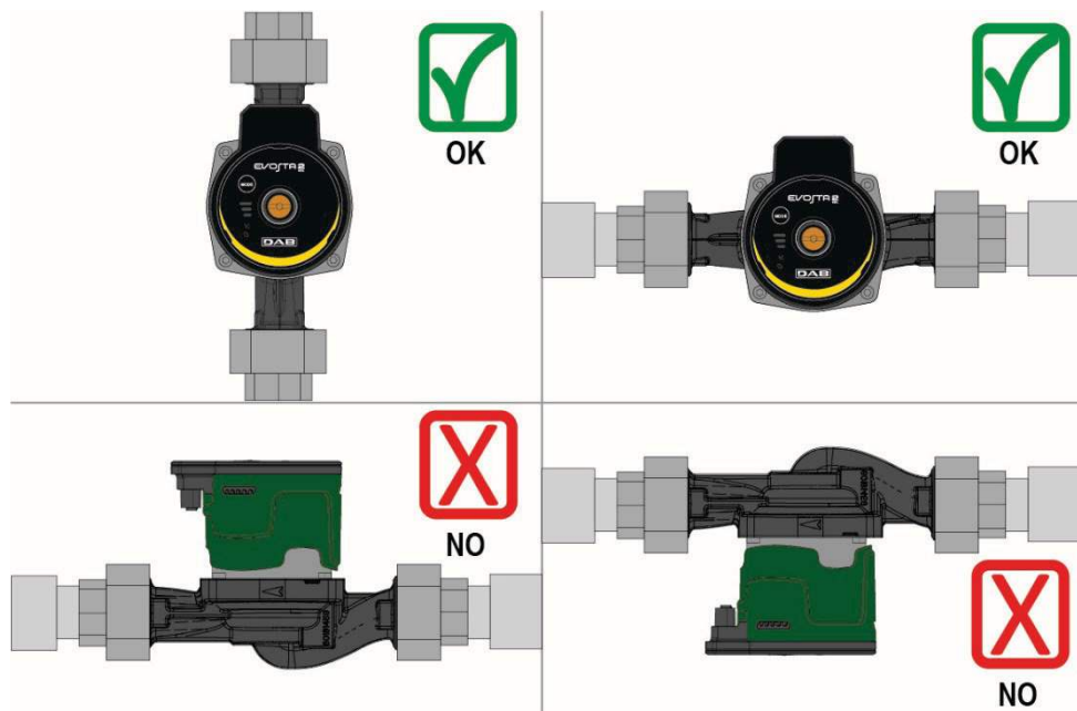
Kuva 12: Asennusasento
