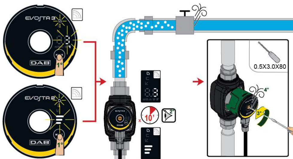
Slika 7: Odzračitev črpalke
