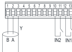
Figur 7: Udtagelig 13-polet klemliste: digitale indgange og MODBUS
