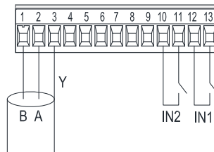
Figura 7: Morsettiere estraibile 13 poli: ingressi digitali e MODBUS
