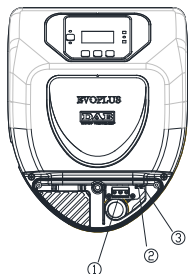
Obr. 4: Elektrické zapojenia (predná strana)
