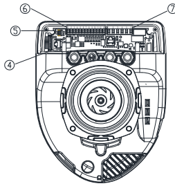
Afbeelding 4: Elektrische aansluitingen (voorzijde) Afbeelding 5: Elektrische aansluitingen (achterzijde)
