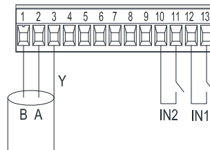
Fig. 7: 13-polig utdragbar kopplingsplint: Digitala ingångar och MODBUS
