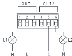
Attēls 9: Iznemams spaļu panelis ar 6 kontaktiem: izeju savienošanas piemērs
