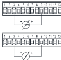
Attēls 8: Iznemams spaļu panelis ar 13 kontaktiem: ieejas 0-10V un PWM
