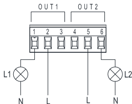
9. ábra : 6 pólusú, kivethető sorkapocs tábla : példa a kimenetek bekötésére
