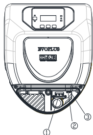
Rys. 4: Podłączenia elektryczne (przód)
