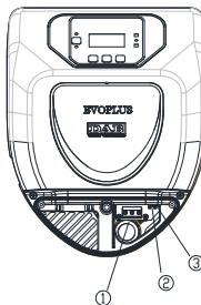
4 pav. Elektros jungtys (priekis)
