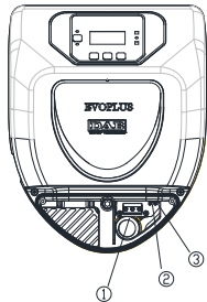
Figura 4: Ligações eléctricas (frente)
