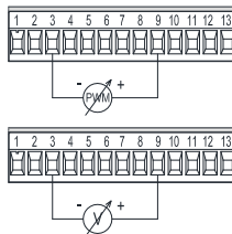
Obr. 8: Vyjimatelná 13 pólová svorkovnice: vstupy 0-10V a PWM
