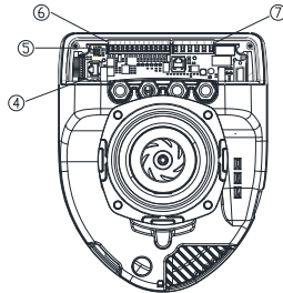
Abbildung 5: Elektroanschlüsse (Rückseite)
