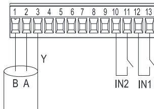
Εικόνα 7: Αφαιρούμενη κλέμια 13 πόλων: ψηφιακές εισόδους και MODBUS
