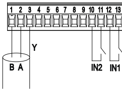
الشكل 7: لوحة طرفية قابلة للإزالة ذات 13 مُقطبًا: المدخلات الرقمية ومدخلات نقل البيانات MODBUS
