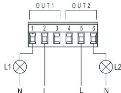
Obr. 9: Vyjimatelná 6 pólová svorkovnice: příklad připojení výstupů
